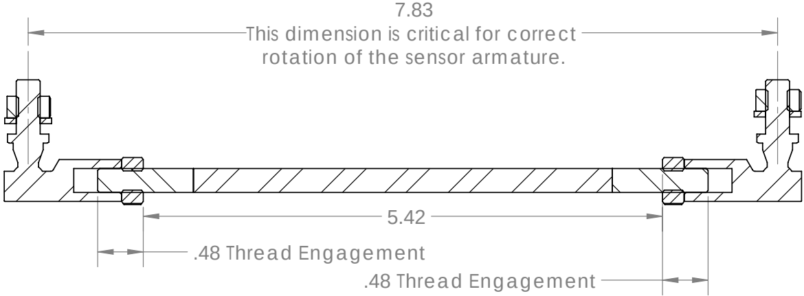
SECTION A-A SCALE 1 : 1.25
