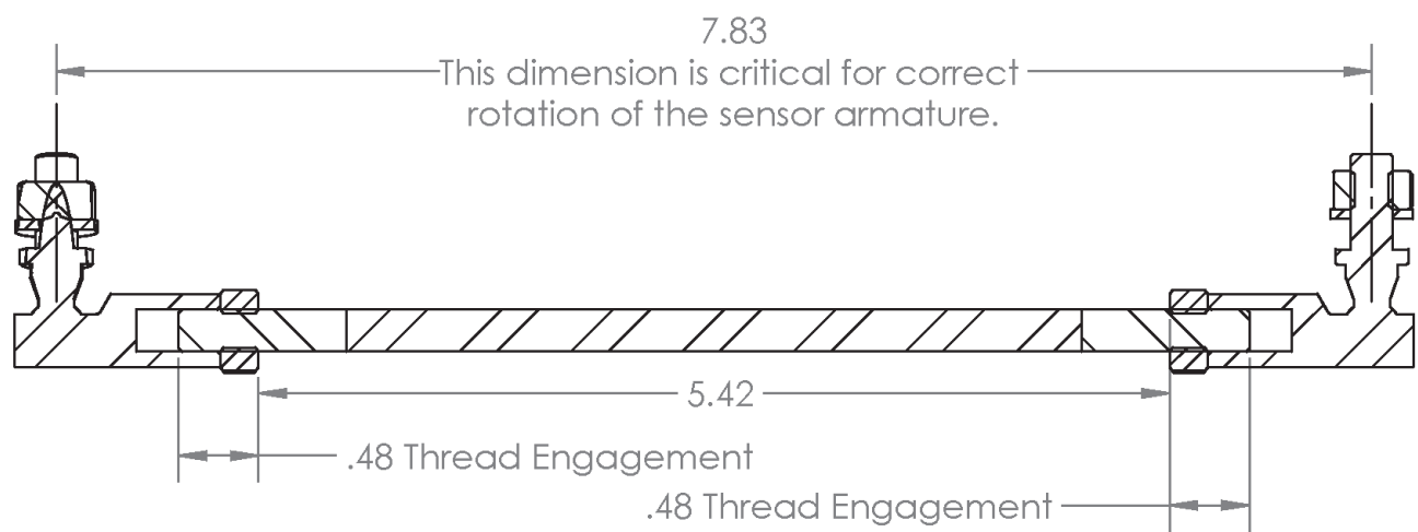
SECTION A-A SCALE 1 : 1.25
