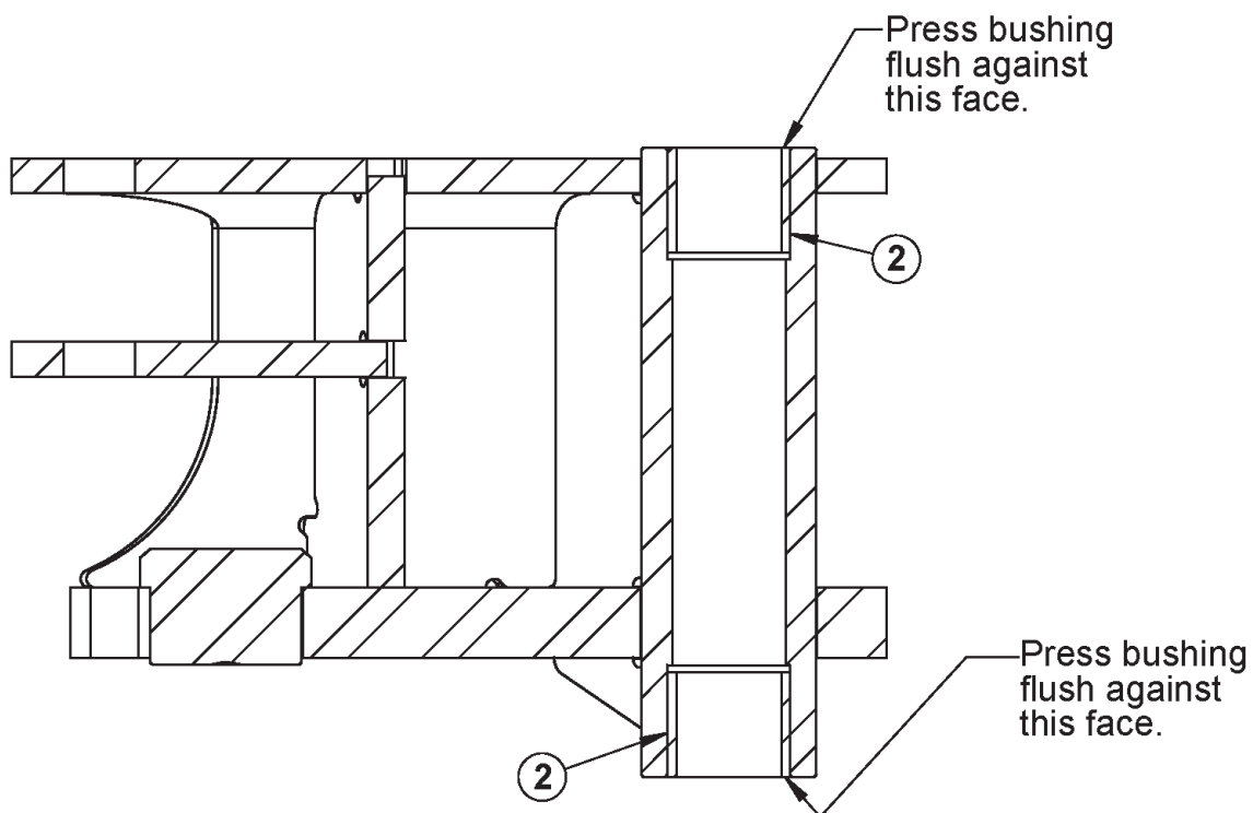
SECTION A-A SCALE 1 : 3
