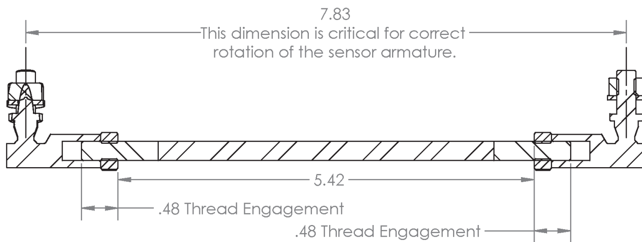
SECTION A-A SCALE 1 : 1.25
